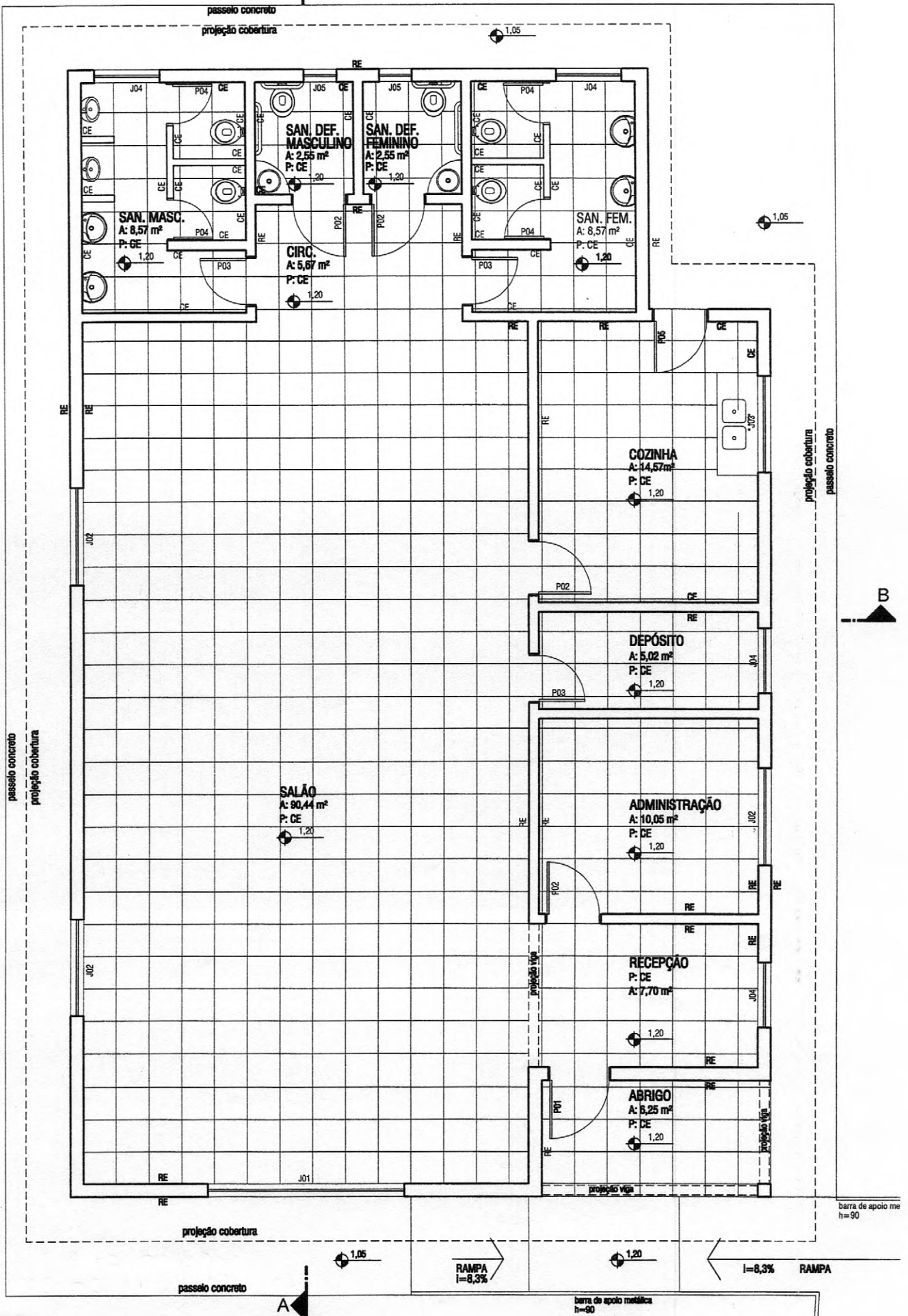
PLANTA BAIXA Sem escala
