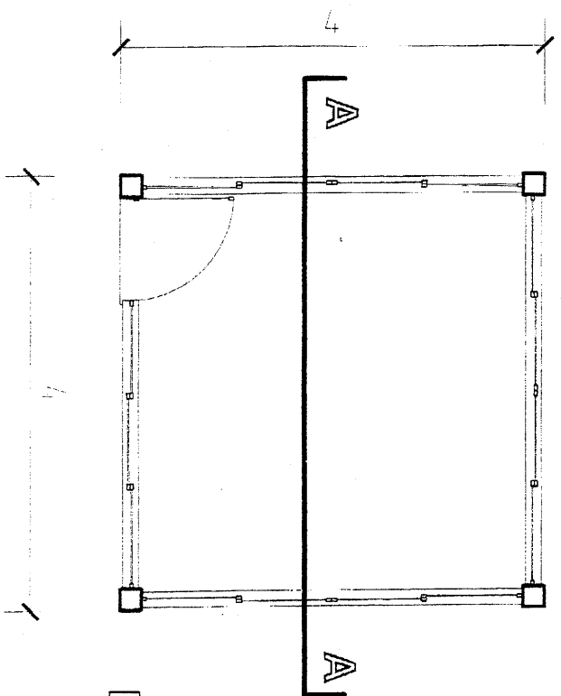
PLANTA BAIXA GUARITA
